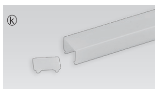
⑫ Square Diffuser HDV-3W-SM HDV-6W-SM HDV-12W-SM HDV-18W-SM HDV-24W-SM 3W 6W 12W 18W 24W
