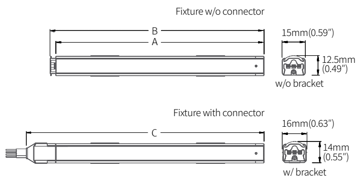
FLX Stix HDV 24W 1123mm(44.21")
