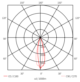
DVS4A 40K-24V-25
