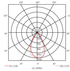
DVS4A 40K-24V-60
