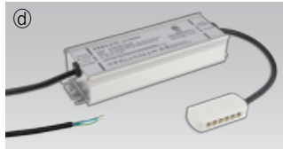
(d) LED Driver : FLC200-24V/T (200W 24V)
